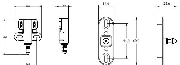
IPLOCK-SCHLIESSBOLZEN 90° KUNSTSTOFF
